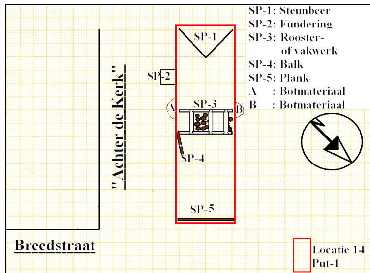
(overzichtstekening)
