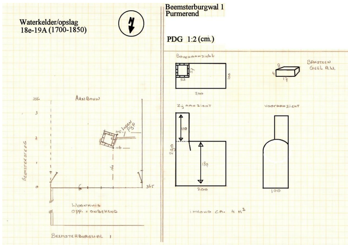
Overzichtstekening van de waterkelder
